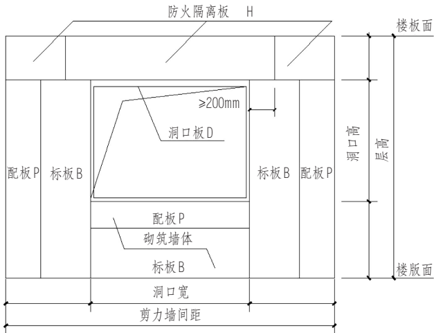
图 6.2.3 复合保温板排版示意图
