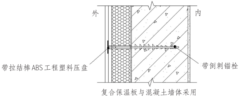
图4.1.5 Ⅲ型锚固装置连接构造
