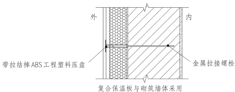
图 4.1.4 II 型锚固装置连接构造
