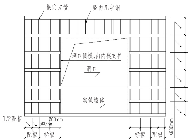
图 6.3.1 轻钢模框组拼立面图
