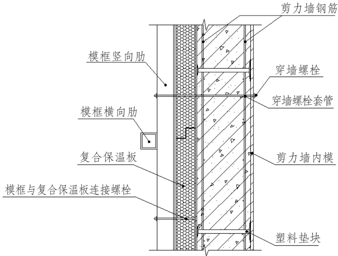
图 6.4.2 复合保温板拼装外模与内模连接示意图
