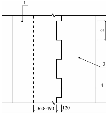
图 5.2.3-3 大直槎
