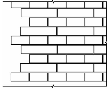
图 5.2.3-2 中直槎
