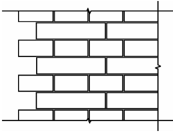
图 5.2.3-1 直槎
